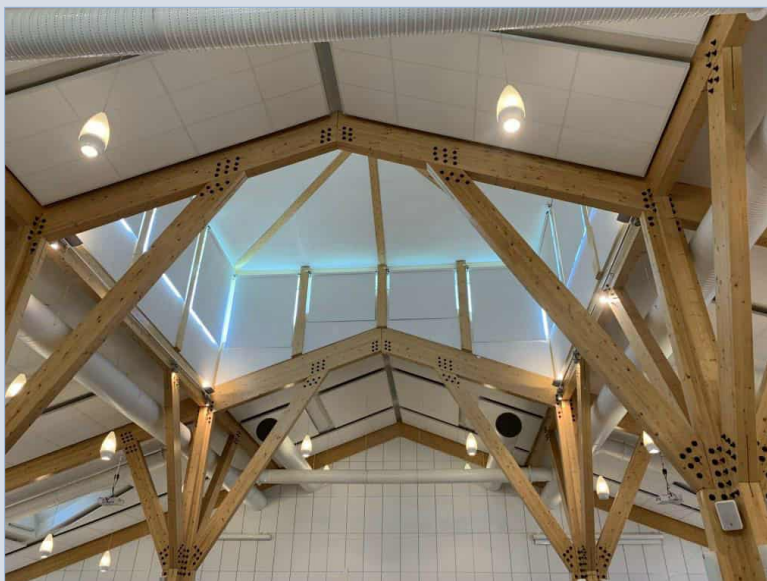
Kattorakenne.
