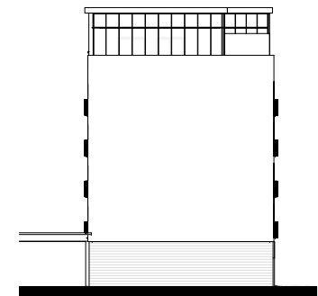
JULKISIVU LÄNTEEN 1 : 500
