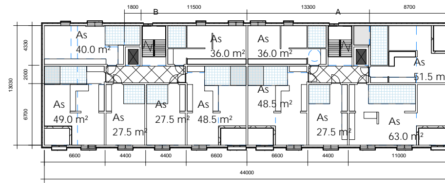
2.-5.KERROS 1 : 400
