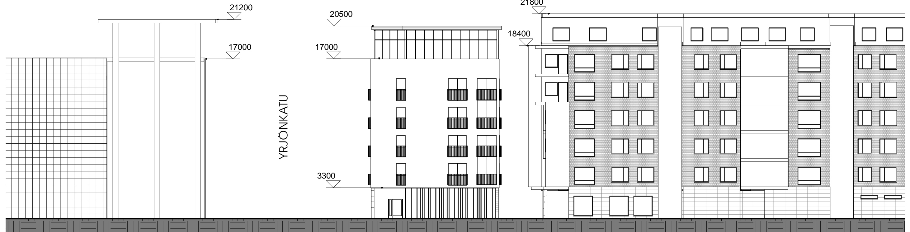
KATUPROJEKTIO MIKONKADULTA 1 : 250
