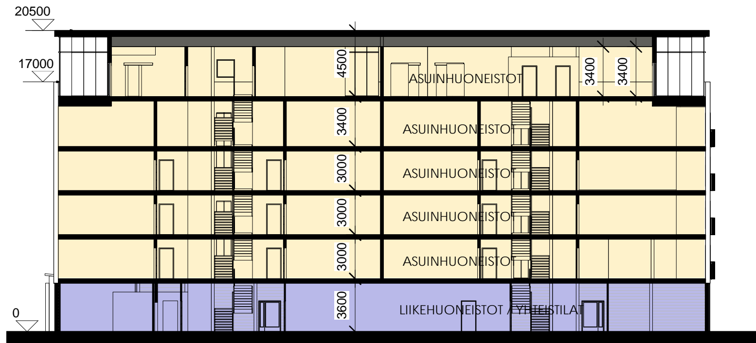
LEIKKAUS A-A 1 : 250
