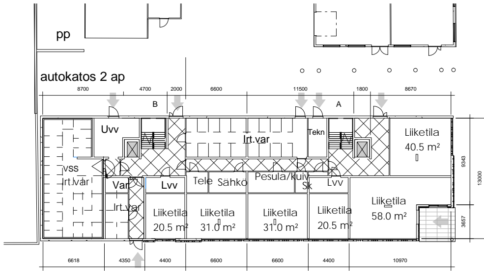
1 KERROS 1 : 400
