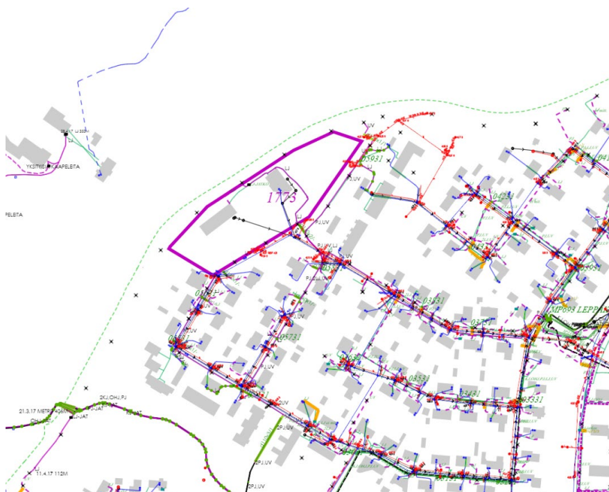
Kuva 5. Ote johtokartasta.
