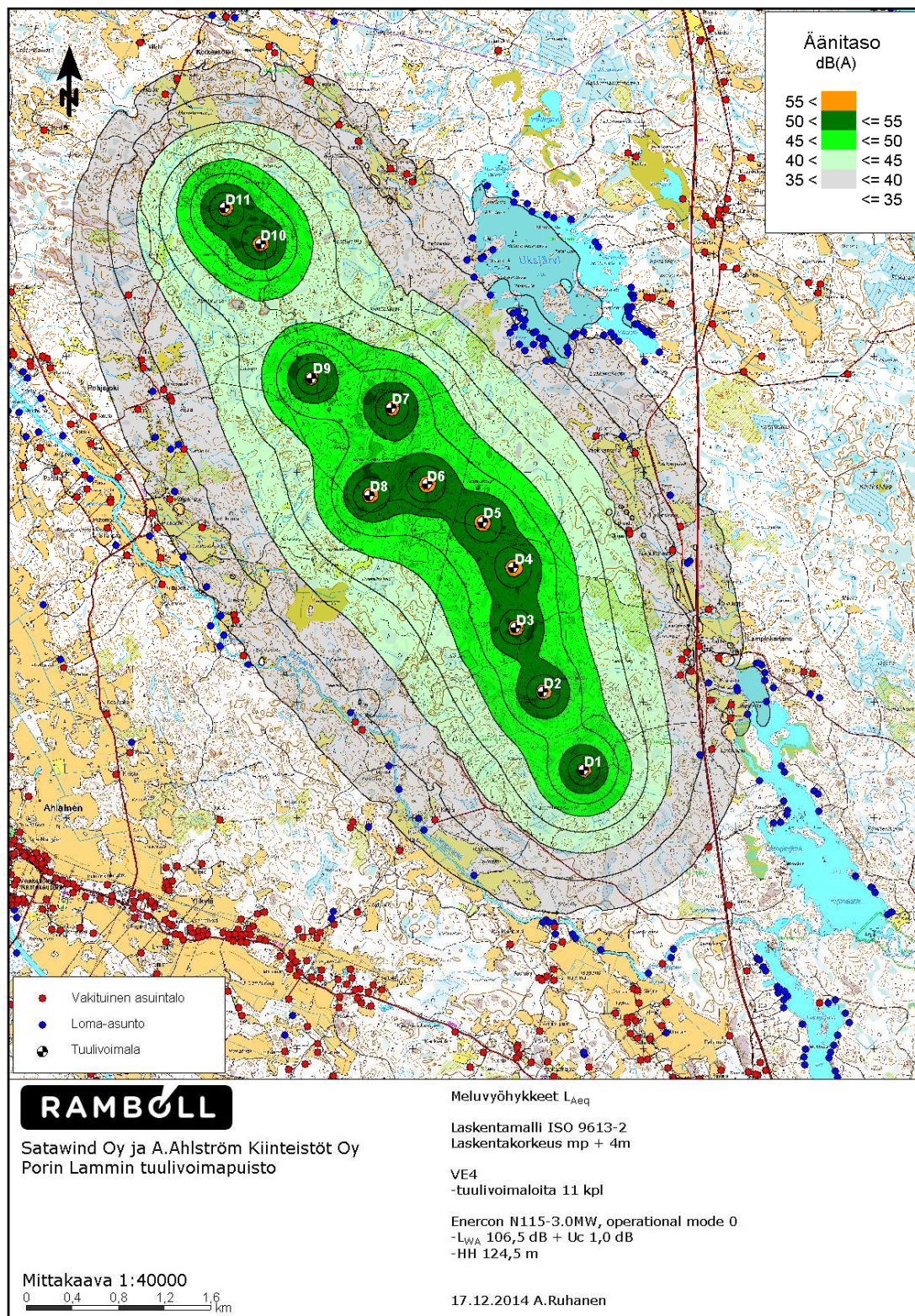
Kuva 17-4. Melumallinnus vaihtoehdossa 4.
