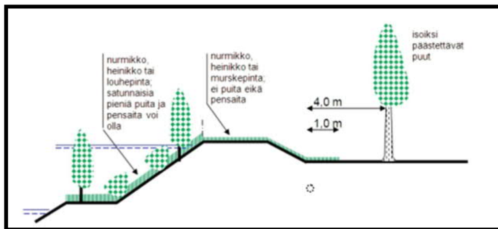
Kuva 26: Pato- turvallisuuden ja padon kunnossa- pidon kannalta sopivat viher- rakentamisen tavat. Porin kaupunki tekninen toimiala.
