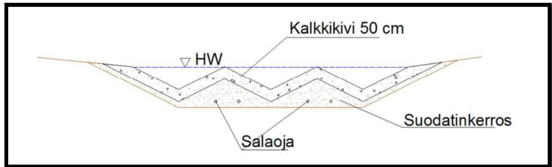
Kuva 14. Pysyväksi rakennetun suotorakenteen periaatepiirros. Ramboll oy.
