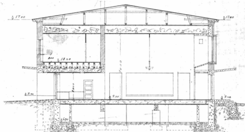
LEIKKAUS C-D
