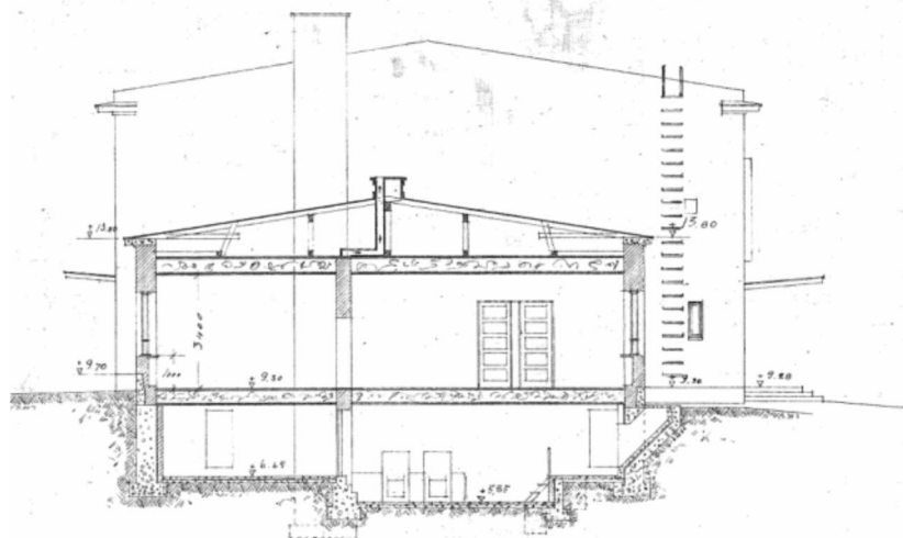
LEIKKAUS A-B
