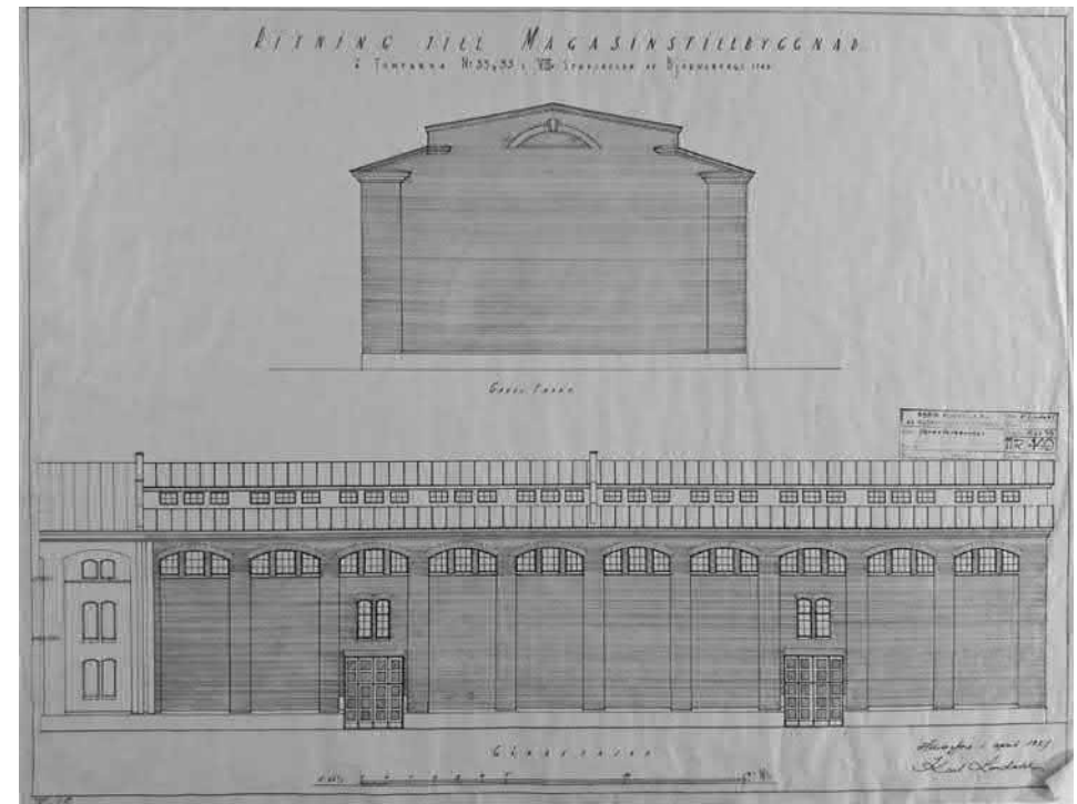
Vuoden 1927 jatko-osan länsijulkisivu ja pohjoispääty, ark. Karl Lindahl. Vasemmalla näkyy vanha osa. Tästä jatko-osasta on nykyisin jäljellä kahden pilarin välinen osa. Sen ikkunat on muurattu ja peitetty sekä säterikatto muutettu. Lähde: Porin Puuvillatehtaan arkisto, Renor Oy, Pori.
