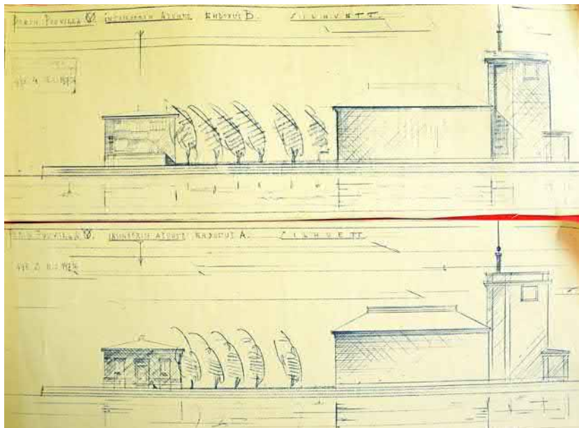
Runar Finnin siluettikuvia, ehdotuksia insinööriasunnoksi 1936. Lähde: Porin Puuvilla-tehtaan arkisto, Renor Oy, Pori.
