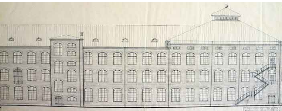
Kehräämmön lisärakennus 1934, sisäpihan julkisivupiirustus. Alkuperäistä julkisivujäsentelyä ja koristelua käytettiin vain pääjulkisivuissa, tehtaan sisäpihan puolelta pilasterit ja hammaslistat puuttuvat. Lisärakennuksen, länsikulman suunnittelusta vastasivat tehtaan rakennusmestarit. Ennen sotaa ehdittiin suunnitella vielä rakennuksen laajennus Koulukadun puolelle, mutta sitä ei toteutettu. Lähde: Porin Puuvillatehtaan arkisto, Renor Oy, Pori.
