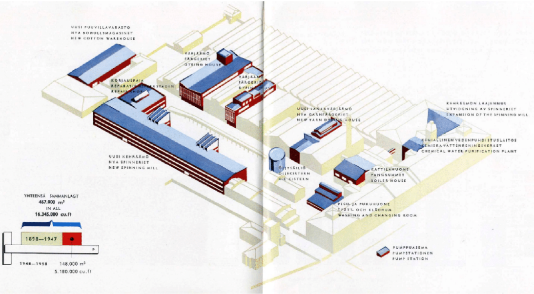
Piirustus tehdasalueen uudisista. Lähde: Zilliacus.
