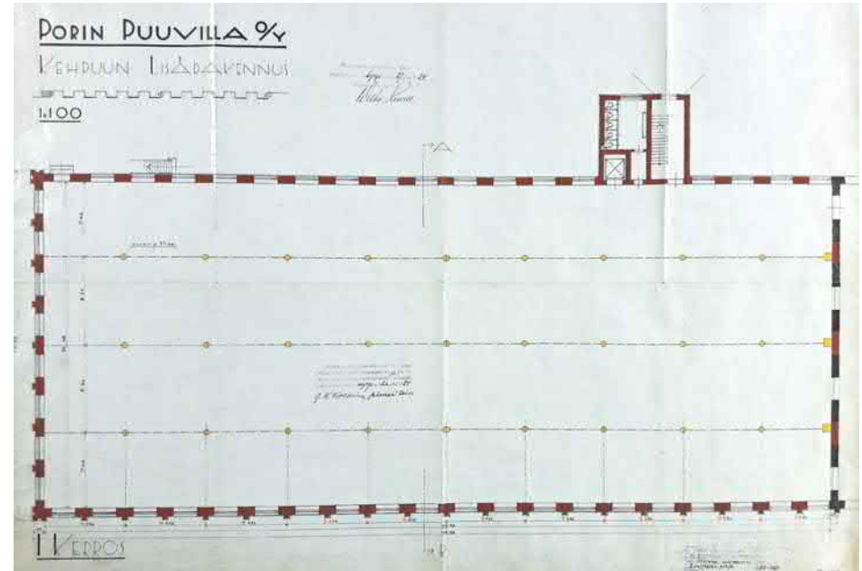
Kehräämmön lisärakennus länteen 1934, 1. krs pohja. Lähde: Digitaaliarkisto/Porin maistraatin arkisto.
