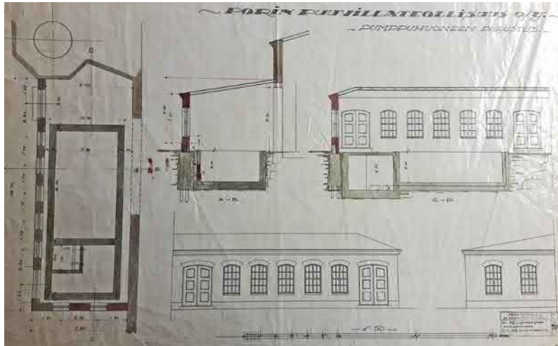
Höyryvoima-aseman pumppuhuoneen laajennuspiirustukset 1920; se sijoittui kattilahuoneen pohjoispuolelle, savupiipun viereen. Lähde: Puuvillatehtaan arkisto, Renor Oy, Pori.
