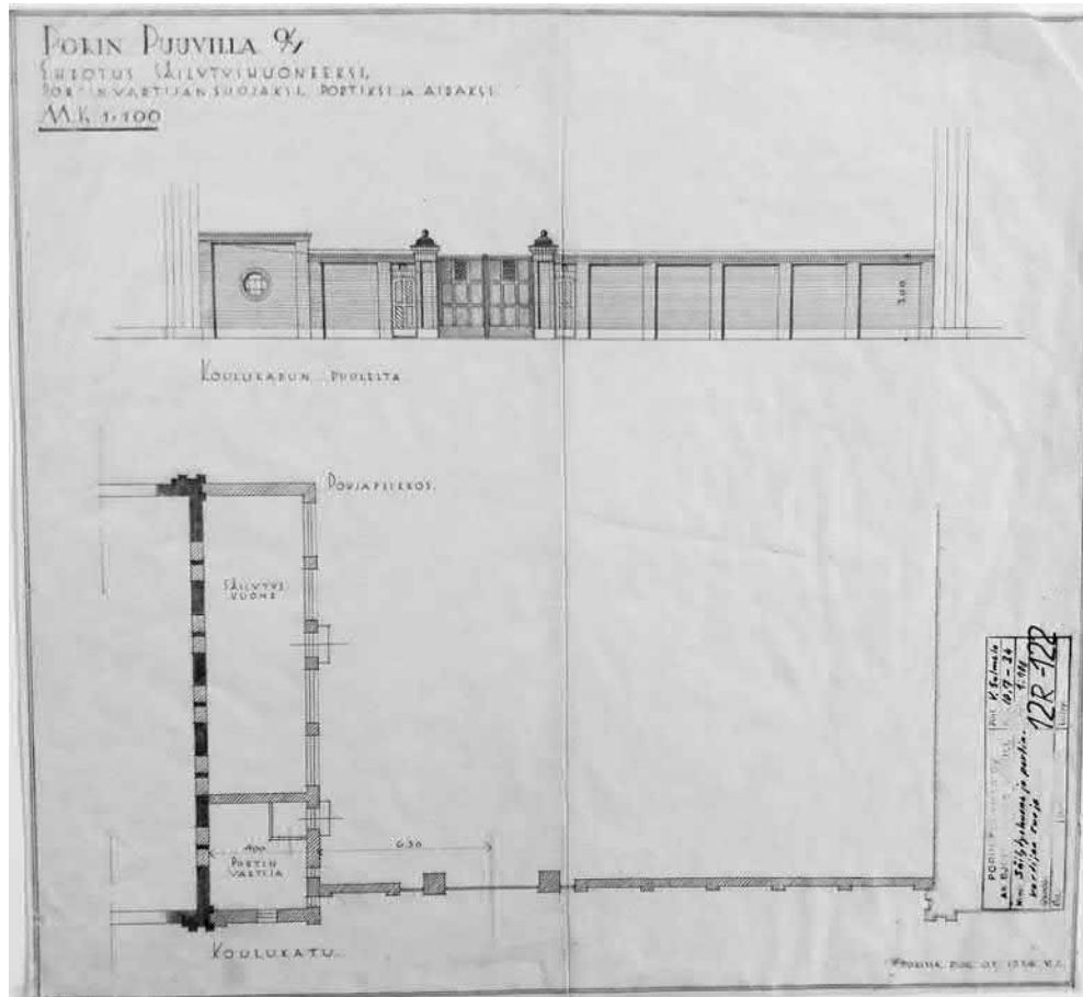
Portinvartijan suoja, säilytyshuone, tehtaan pääportti sekä aita vuoden 1934 suunnitelmassa. Ei tietoa toteutuivatko portti ja muuri, myöhemmin paikalla oli teräskaarinen porttiosa. Suunnitelman laati rkm Väinö Salmela. Lähde: Porin Puuvillatehtaan arkisto, Renor Oy, Pori.
