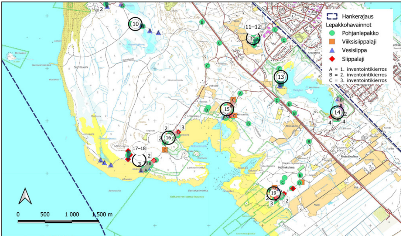
Kuva 5. Lepakkohavainnot inventointikierrroksittain ja arvokkaat lepakkoalueet. Indeksikartta saattaa sisältää useamman kuin yhden arvoalueen. Havainnoissa on merkitty yksilömäärä ainoastaan, mikäli se on vähintään kaksi yksilöä. Ilman merkintää olevat koskevat yhtä yksilöä.
