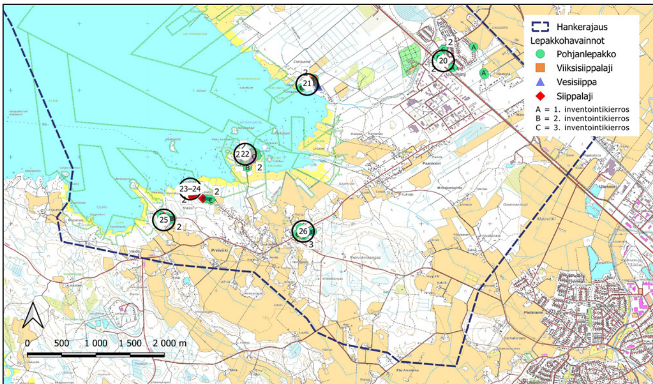
Kuva 6. Lepakkohavainnot inventointikierrroksittain ja arvokkaat lepakkoalueet. Indeksikartta saattaa sisältää useamman kuin yhden arvoalueen. Havainnoissa on merkitty yksilömäärä ainoastaan, mikäli se on vähintään kaksi yksilöä. Ilman merkintää olevat koskevat yhtä yksilöä.
