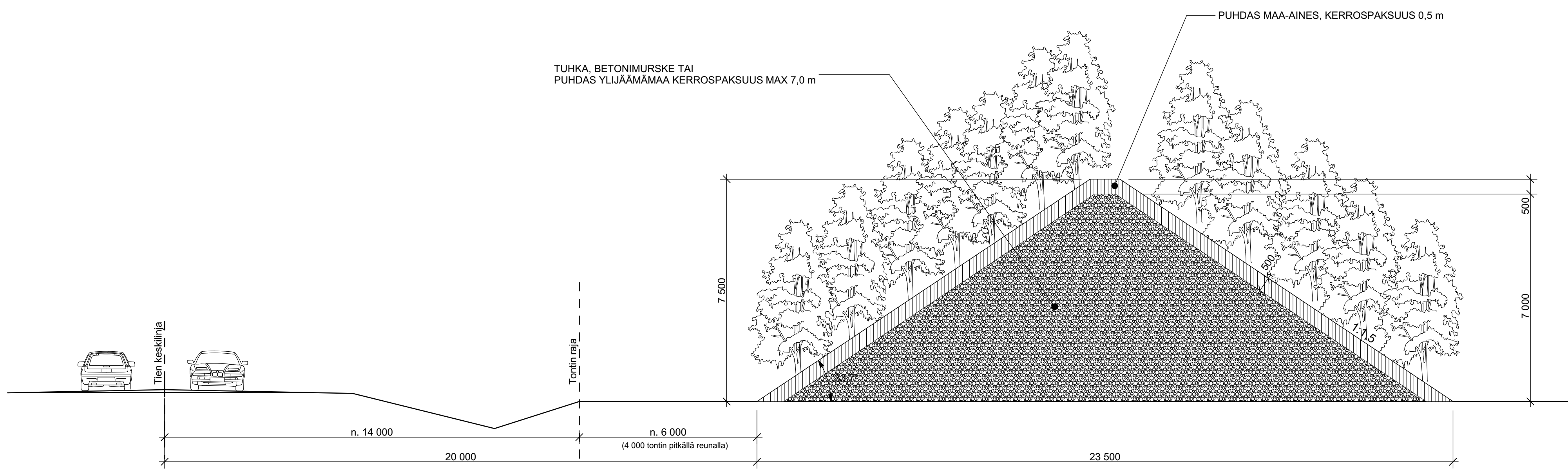
LEIKKAUS, 7,5 m KORKEA MELUVALLI
