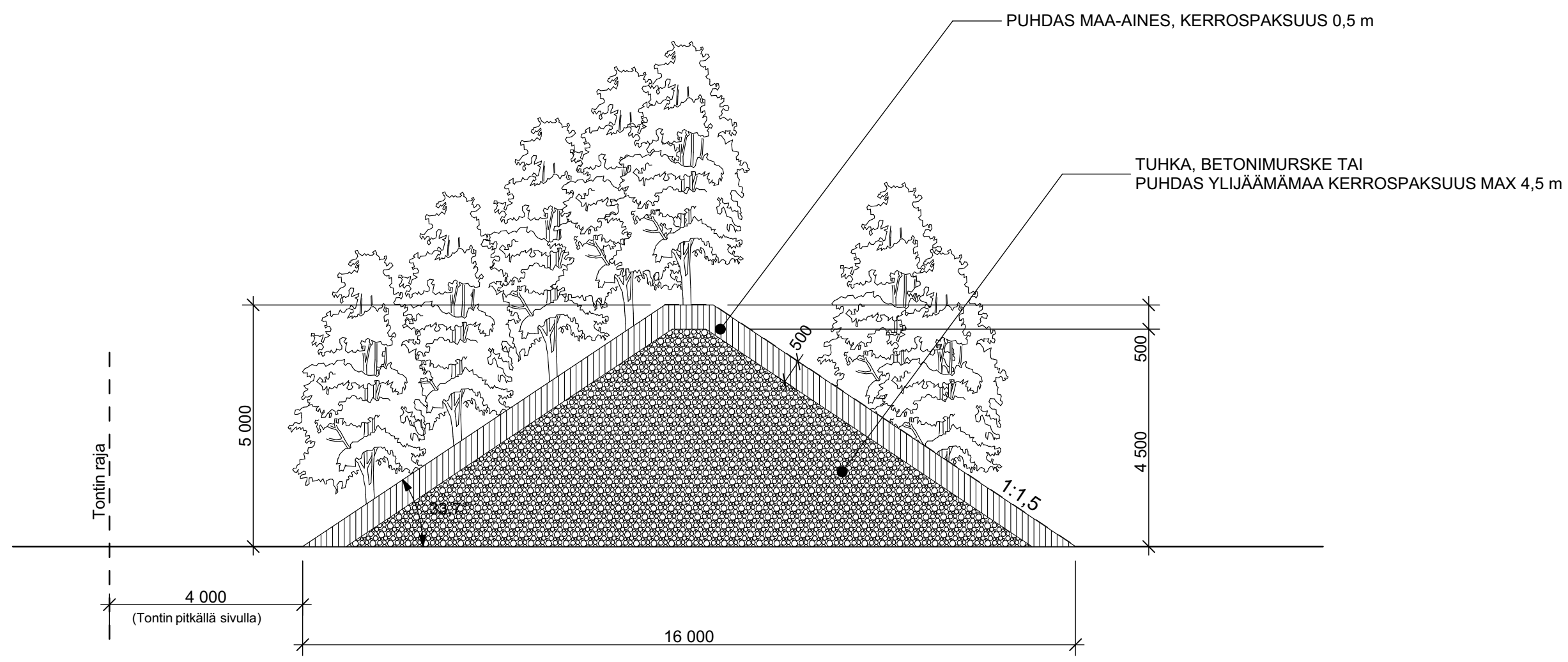
LEIKKAUS, 5 m KORKEA MELUVALLI
